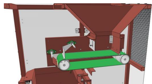
Förderband mit Schichthöhenbegrenzer
