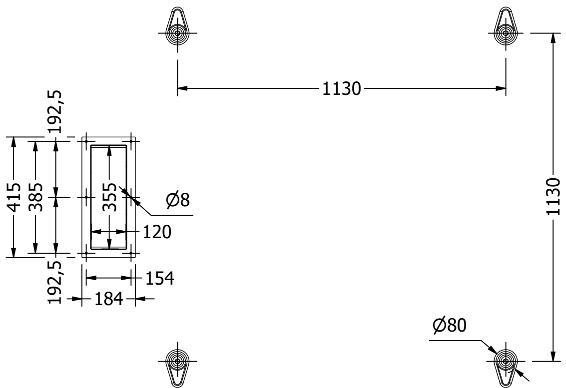
B-B ( 1 : 15 )
